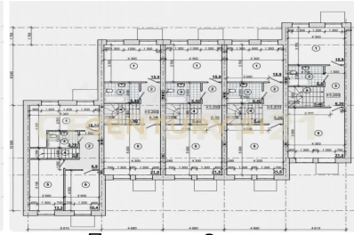
План дома 2 этажа
