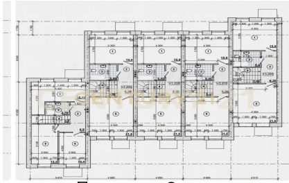
План дома 2 этажа
